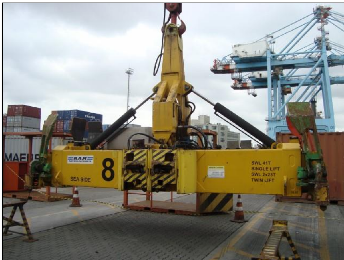
Figura 1. Spreader automático, SPR-08.
